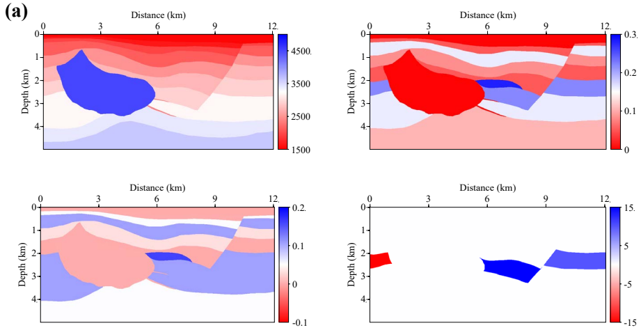
Figure 6 The anisotropy parameters of Hess TTI model. (a) V_p , (b) \epsilon , (c) \delta , (d) \theta .
